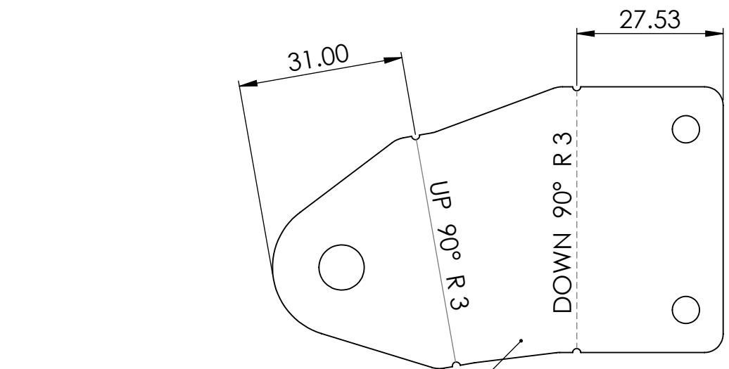
GSB-03 v1.0L, SM-FLAT-PATTERN
